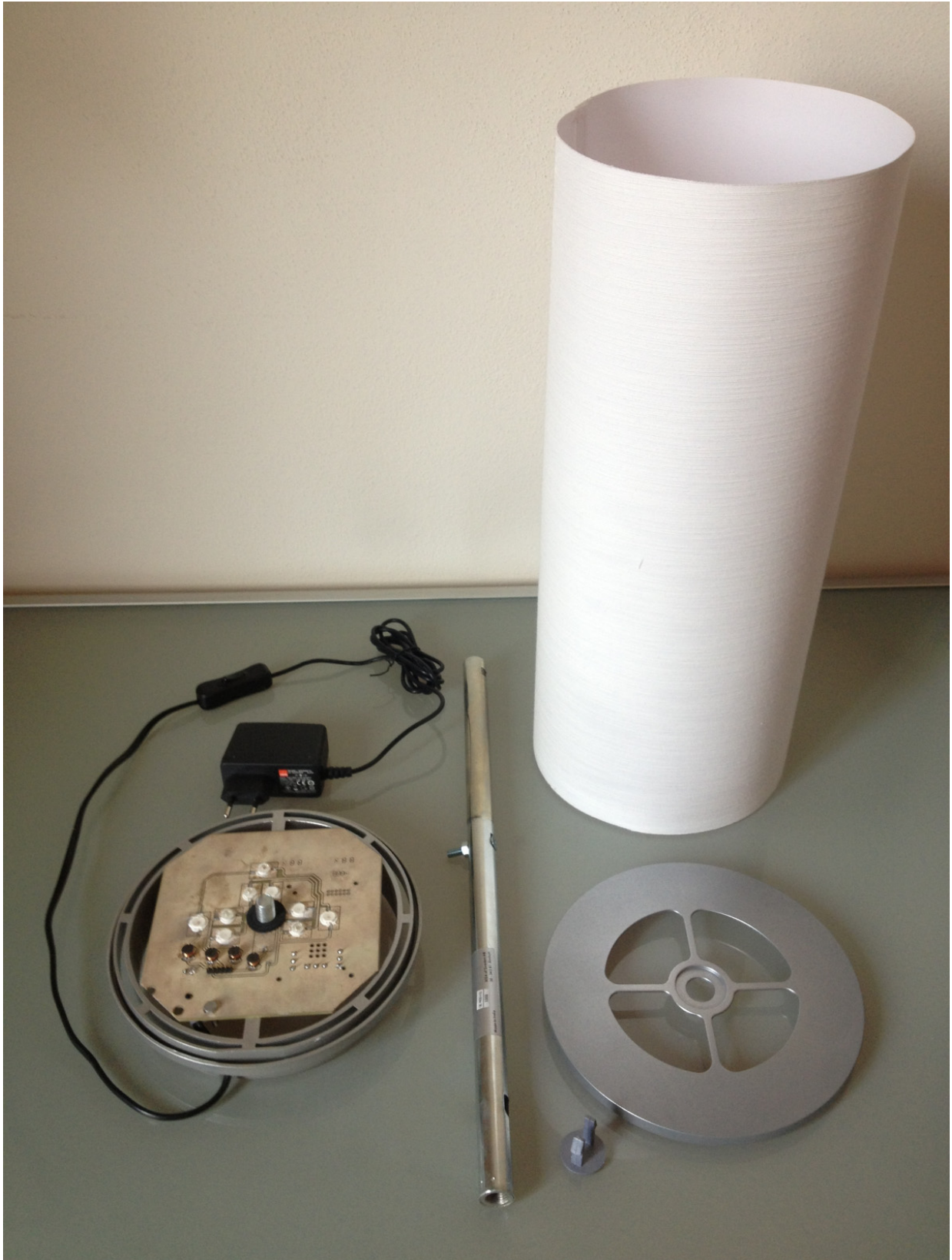
Figura 1 – Componenti Vidja-POWERino
